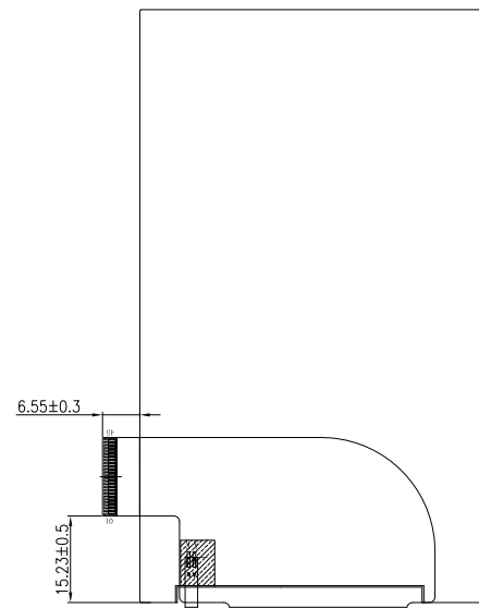
FPC弯折示意图 弯折出货
